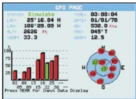
Fig. 7.1 - La pagina GPS
