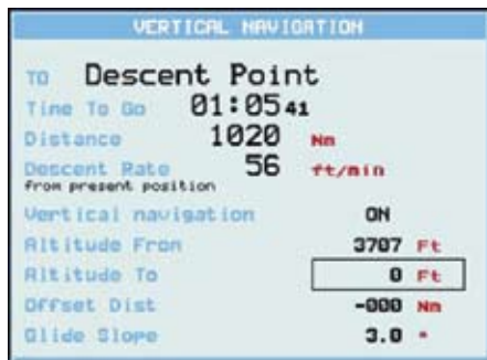
Fig. 10.4 - Pagina Navigazione Verticale
