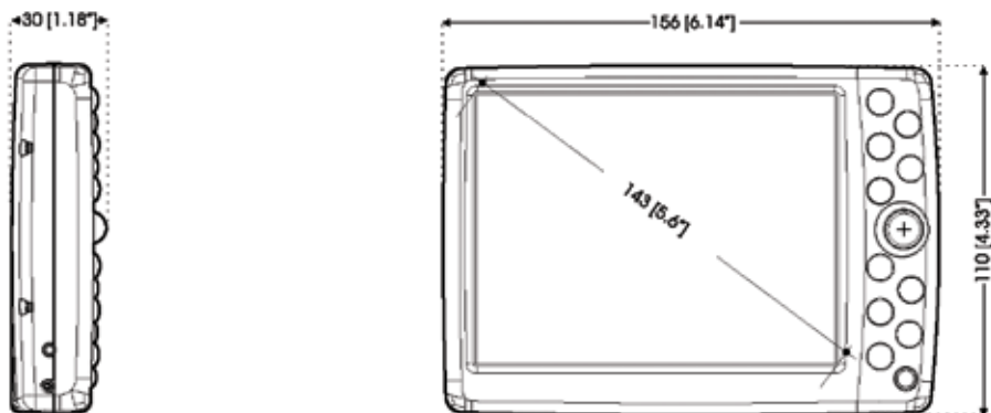
Fig. 15.4 - Dimensioni del GEOPILOT
