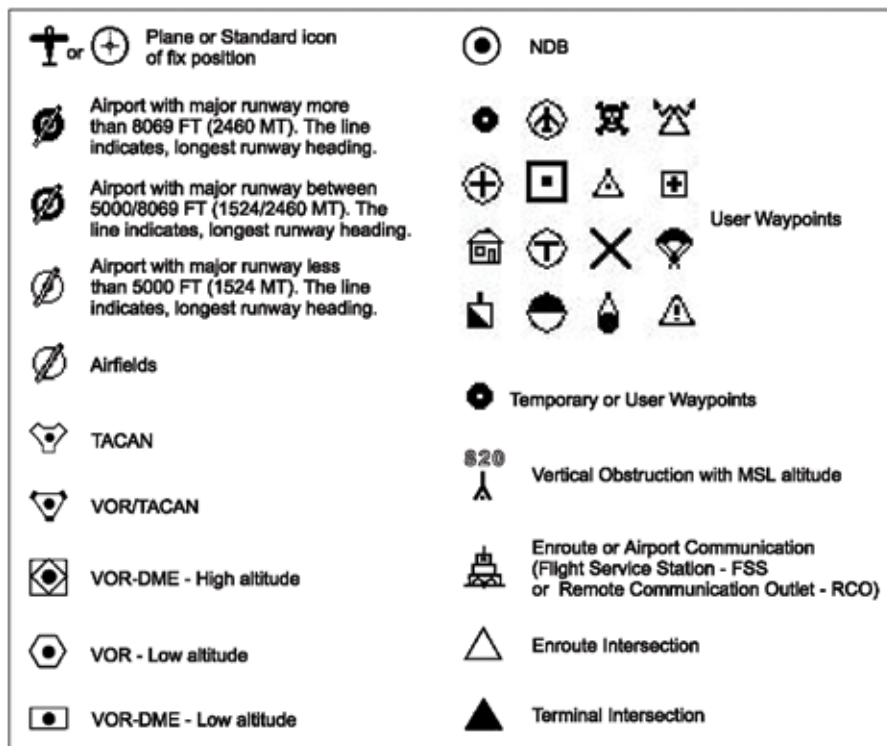
Fig. 1.3.4 - Icone Mappa
