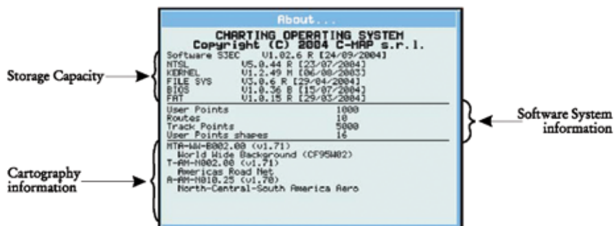
Fig. 15.4.4 - Pagina Informazioni
