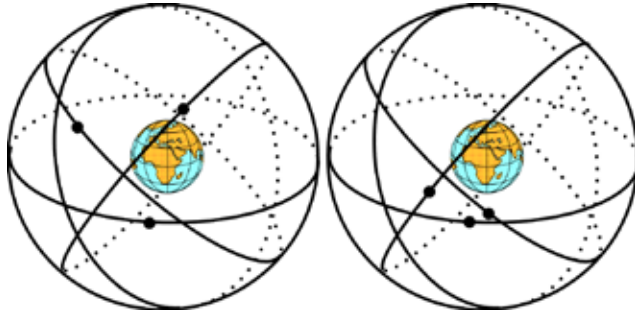
Fig. 7.2.1 - HDOP
