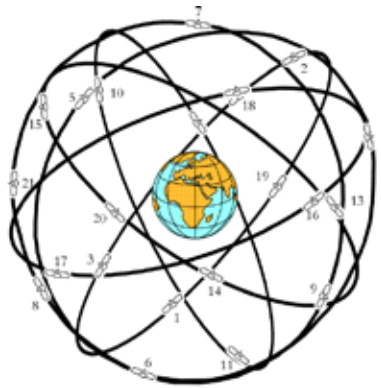
Fig. 7.2 - Costellazione GPS
